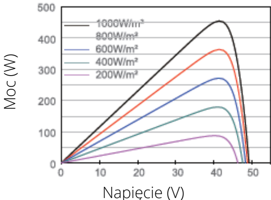
Krzywa Moc - Napięcie JAM72S20-455/MR
