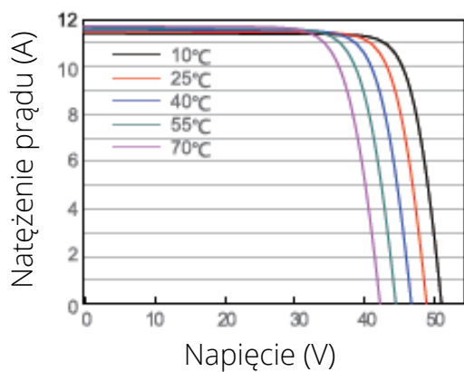
Krzywa Prąd - Napięcie JAM72S20-455/MR
